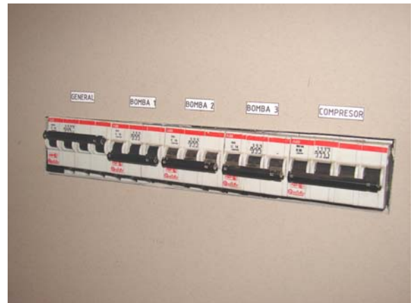
Figura3: Vista de la instalación eléctrica realizada sobre bandejas y de los tableros con sus correspondientes llaves térmicas y disyuntor en el Laboratorio de Máquinas Térmicas.
